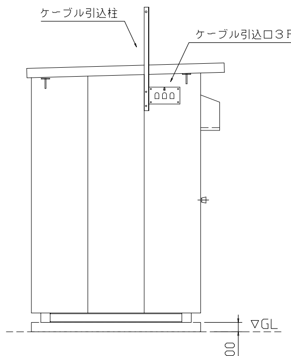
立面図 D S=1/40
