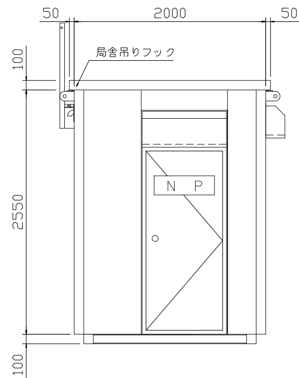
立面図 A S=1/40
