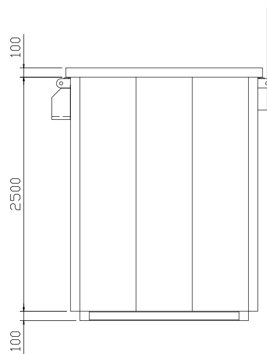
立面図 C S=1/40
