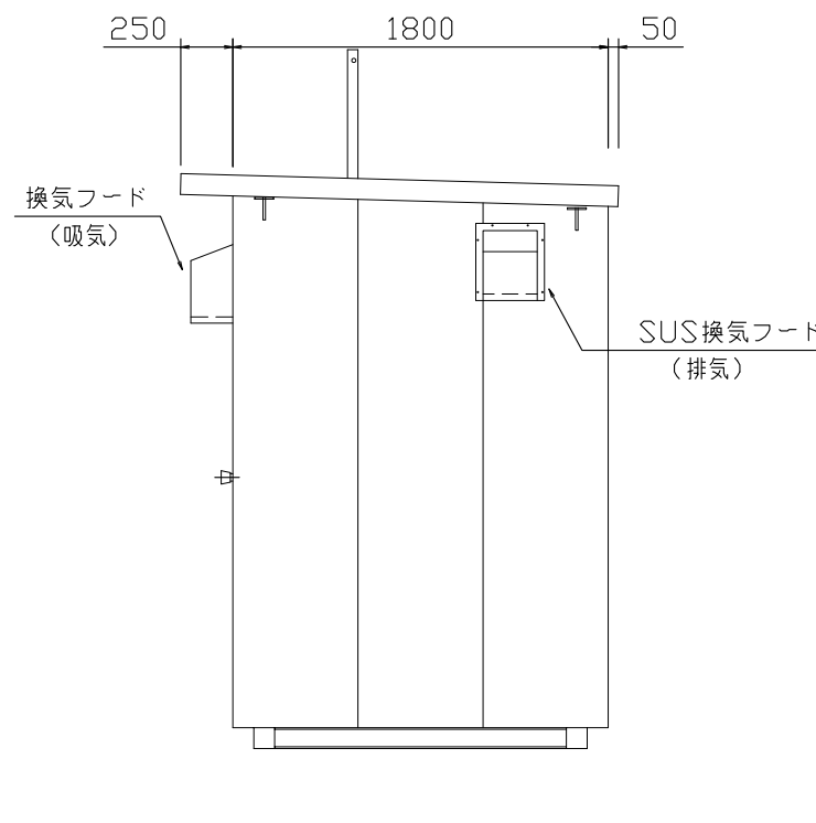
立面図 B S=1/40
